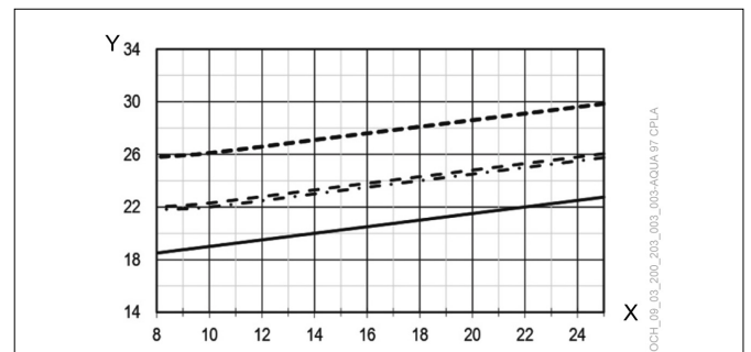
X Wassertemperatur [°C] Y Leistungsaufnahme [kW]
